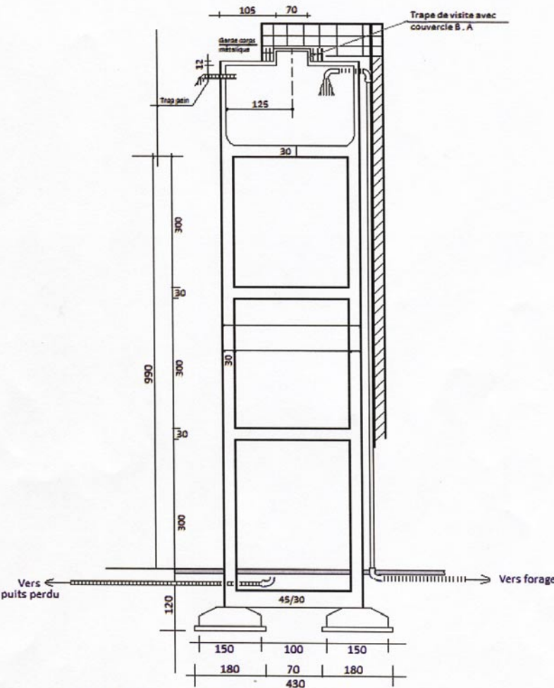
COUPE VERTICALE SUR CHATEAU D'EAU DE 10 m 3 SUS 9m SOUS CUVE
